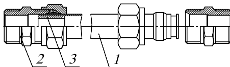
Рис.7. Соединение нагревательных элементов конвектора.
