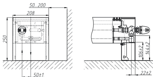
HKOH1,5 Pro 10-15.050...250 T2 П
